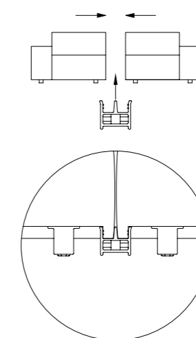
Cuciture elemento terminale. Il terminale sulla seduta ha una parte curva. In composizione l'elemento va agganciato dal lato indicato dalla freccia
